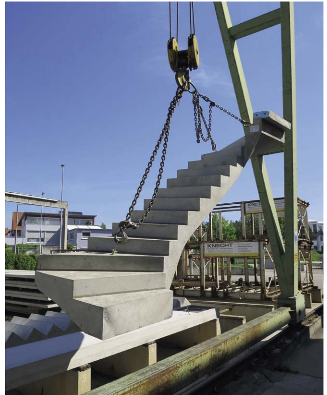
Abb. 7.2: Betonfertigteiltreppen sind direkt nach der Montage begehbar.
