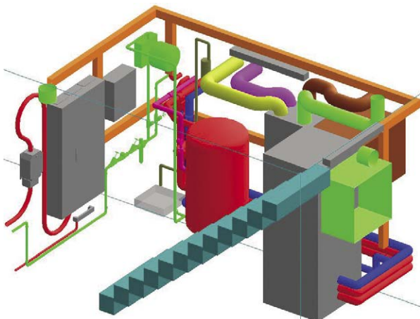
Abb. 13.6: Die Raumzellen in Betonfertigteilbauweise konzentrieren die Technische Gebäudeausrüstung auf einen Raum mit komfortablen Wartungsmöglichkeiten.
